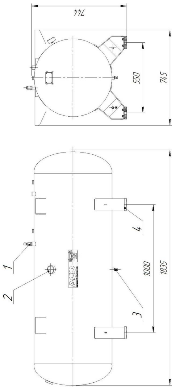
Рисунок 3. Ресивер 1 – клапан предохранительный, 2 – манометр, 3 – пробка сливная, 4 – подушка амортизационная
